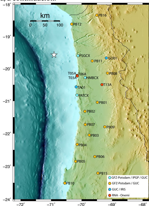
Figura 1: Mapa topográfico con las estaciones que componen la red IPOC y RNA; el color marca la procedencia de la estación, según la escala del borde inferior derecho. La estrella blanca marca el epicentro del terremoto 1 de abril de 2014. La localización exacta de cada estación se presenta en el Anexo.
